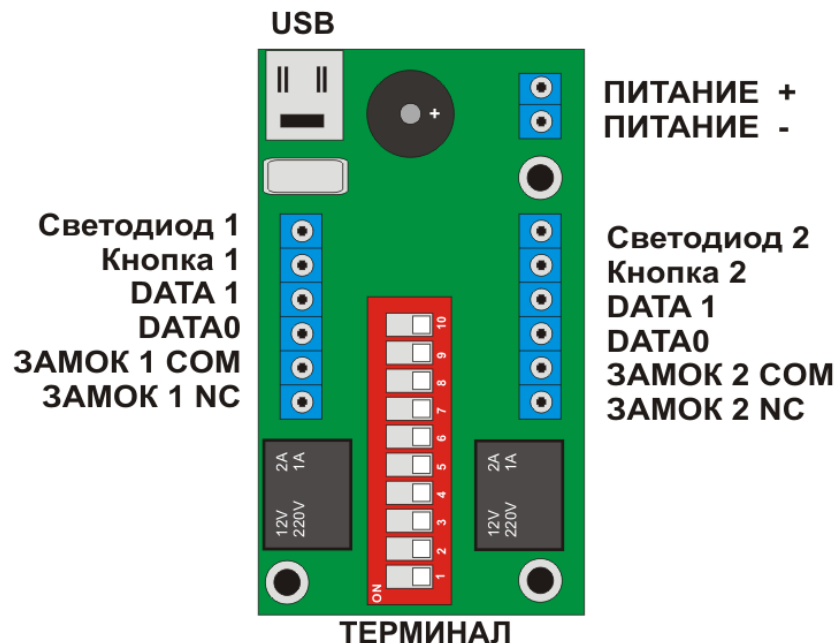
Рис.1 Зовнішній вигляд та підключення пристрою
